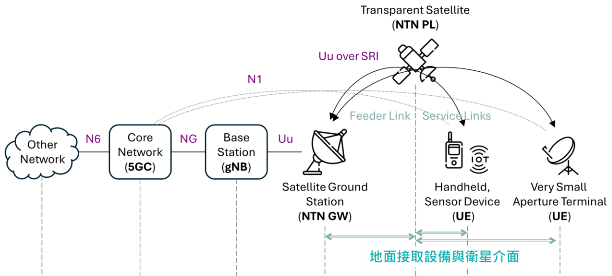
圖 23、3GPP NTN 通透型系統的地面接取設備與衛星介面
