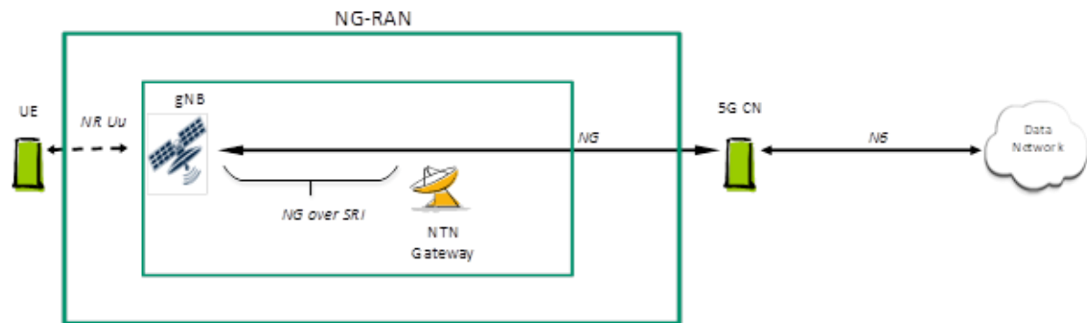
圖 8、3GPP NTN 再生型系統架構
