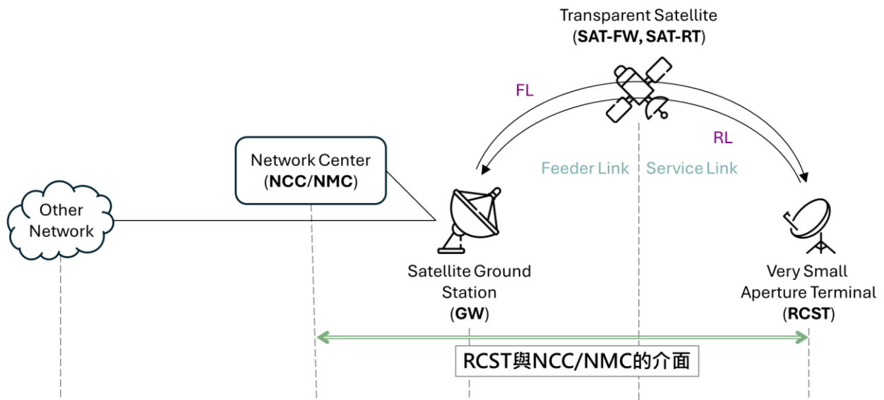
圖 40、DVB-S/RCS 通透型系統的 RCST 與 NCC/NMC 的介面
