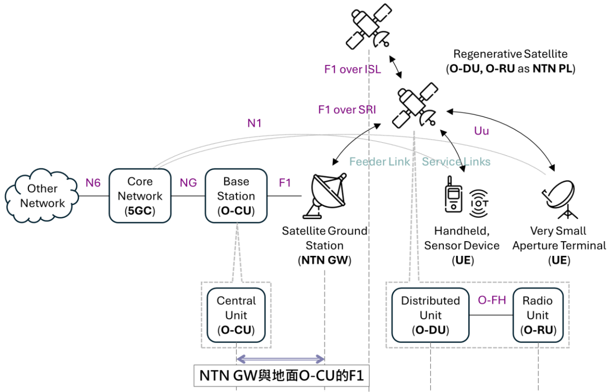
圖 62、3GPP NTN 再生型系統 O-RAN 的 NTN GW 與地面 O-CU 的 F1
