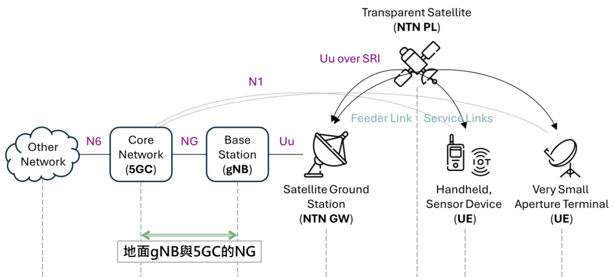
圖 42、3GPP NTN 通透型系統的地面 gNB 與 5GC 的 NG
