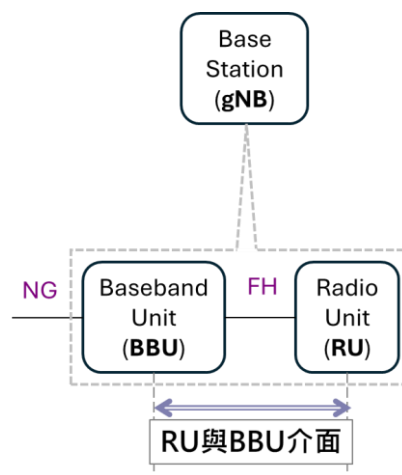
圖 53、3GPP RAN 的 RU 與 BBU 的介面
