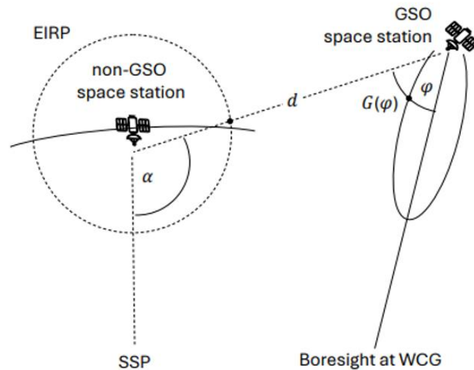
圖 33、規範衛星間方向干擾的 EPFD 示意
