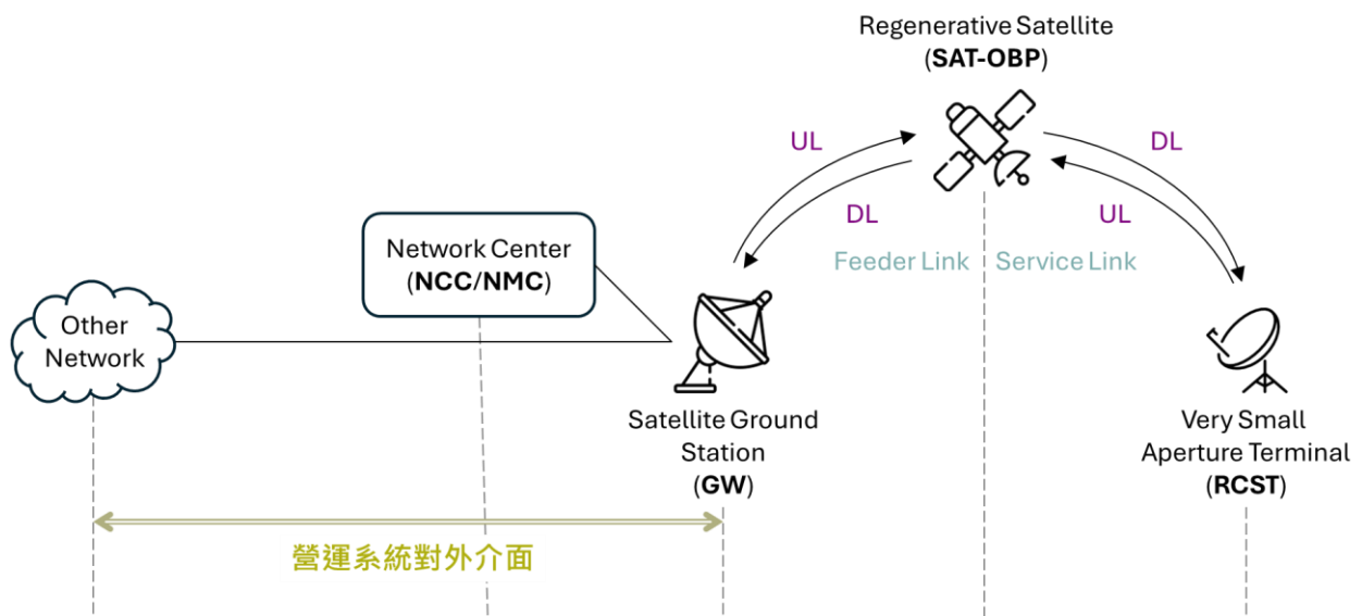
圖 14、DVB-S/RCS 再生型系統的營運系統對外介面
