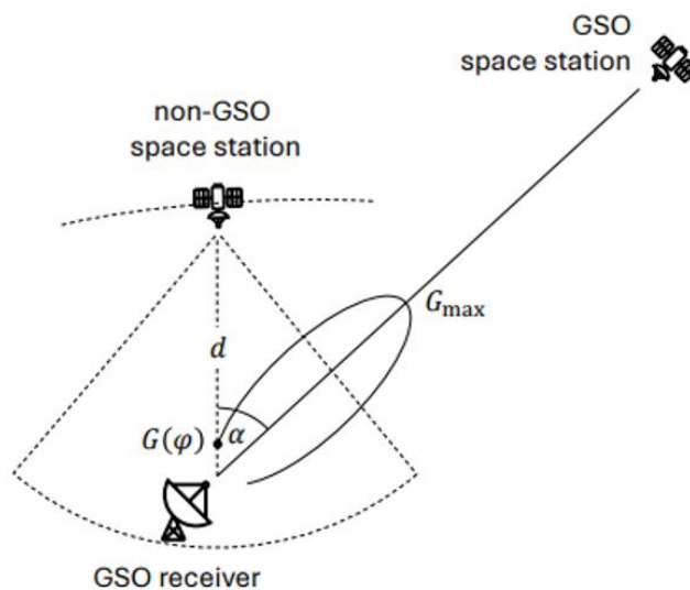
圖 31、規範下行方向干擾的 EPFD 示意
