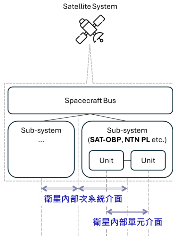
圖 27、衛星內部次系統/單元介面
