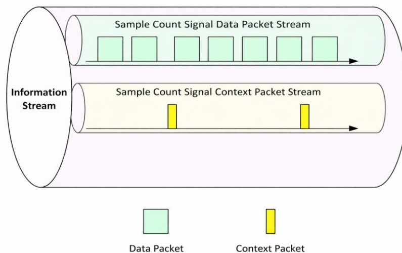
圖 52、DIFI v1.3.0 雙封包機制的架構示意
