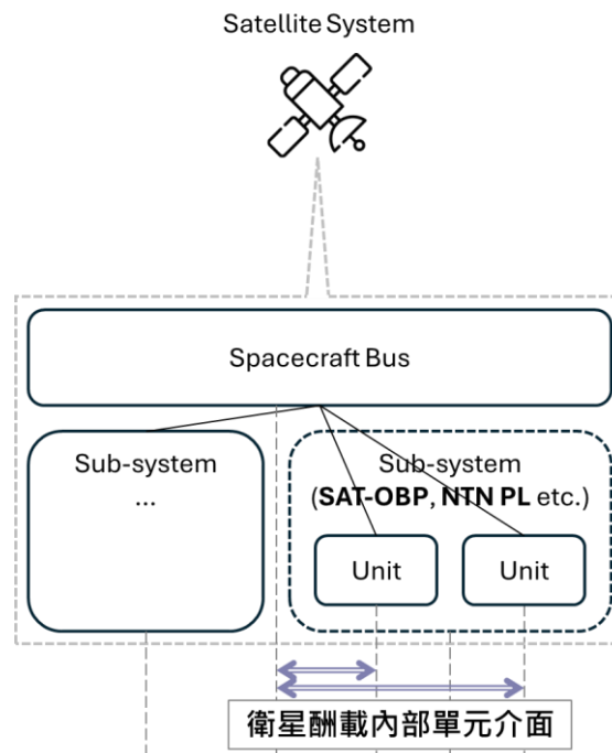
圖 55、與本體 (BUS) 共用的衛星酬載內部單元介面
