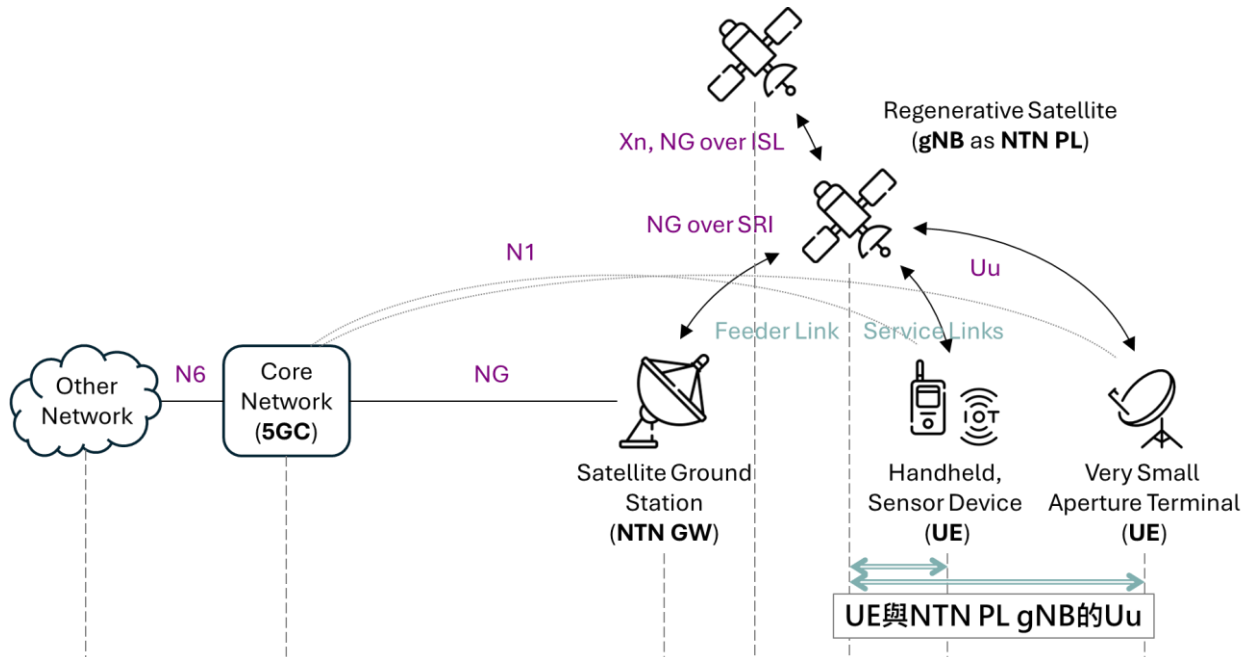
圖 48、3GPP NTN 再生型系統的 UE 與 NTN PL gNB 的 Uu
