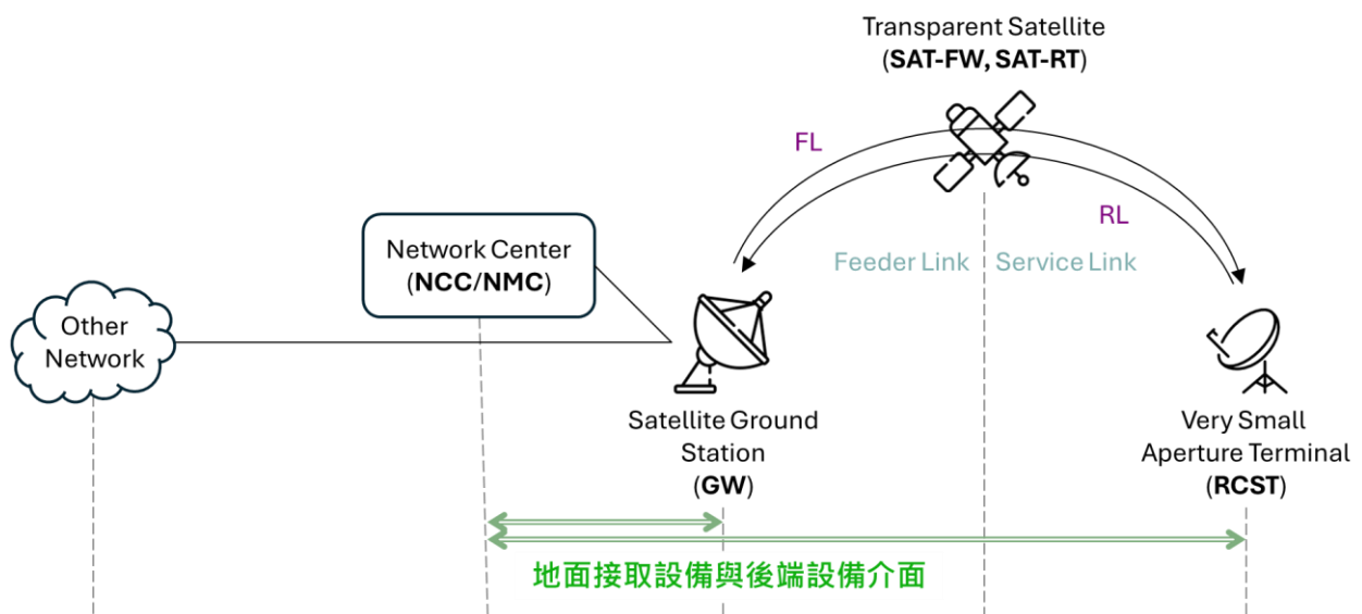
圖 17、DVB-S/RCS 通透型系統的地面接取設備與後端設備介面
