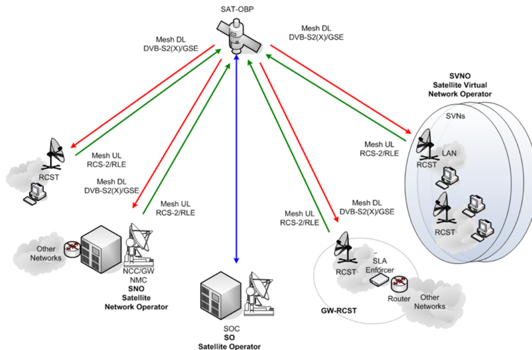
圖 4、DVB-S/RCS 再生型系統架構
