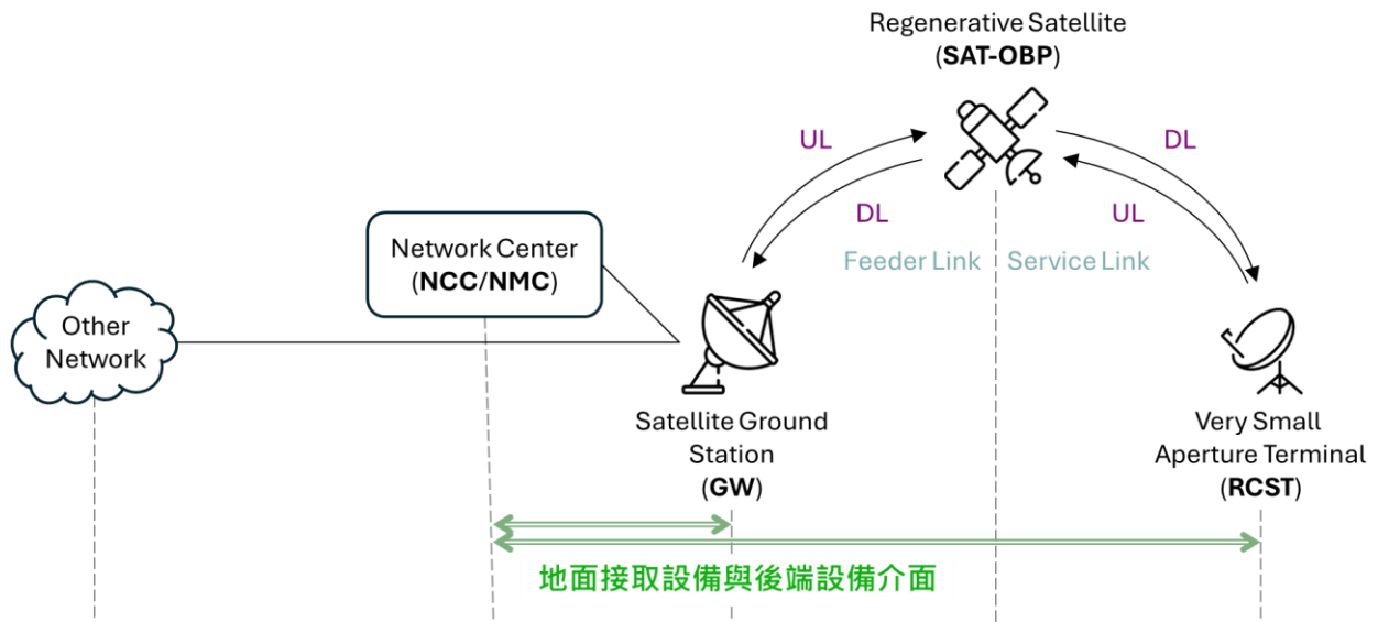
圖 18、DVB-S/RCS 再生型系統的地面接取設備與後端設備介面
