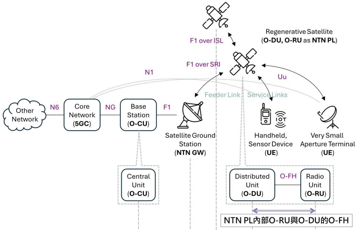
圖 59、3GPP NTN 再生型系統 O-RAN 的 NTN PL 內部 O-RU 與 O-DU 的 O-FH
