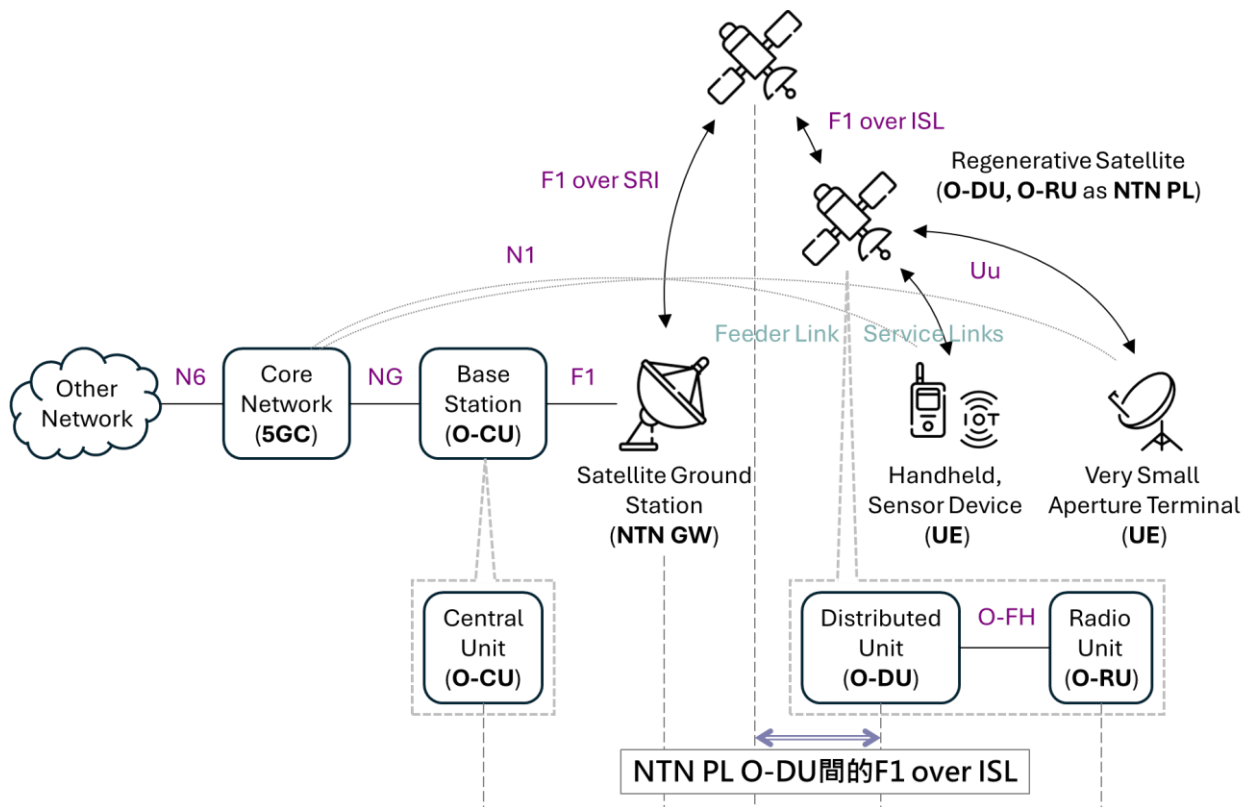
圖 60、3GPP NTN 再生型系統 O-RAN 的 NTN PL O-DU 間的 F1 over ISL
