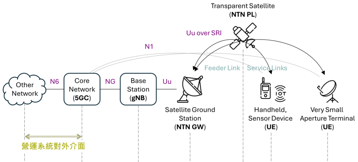
圖 15、3GPP NTN 通透型系統的營運系統對外介面
