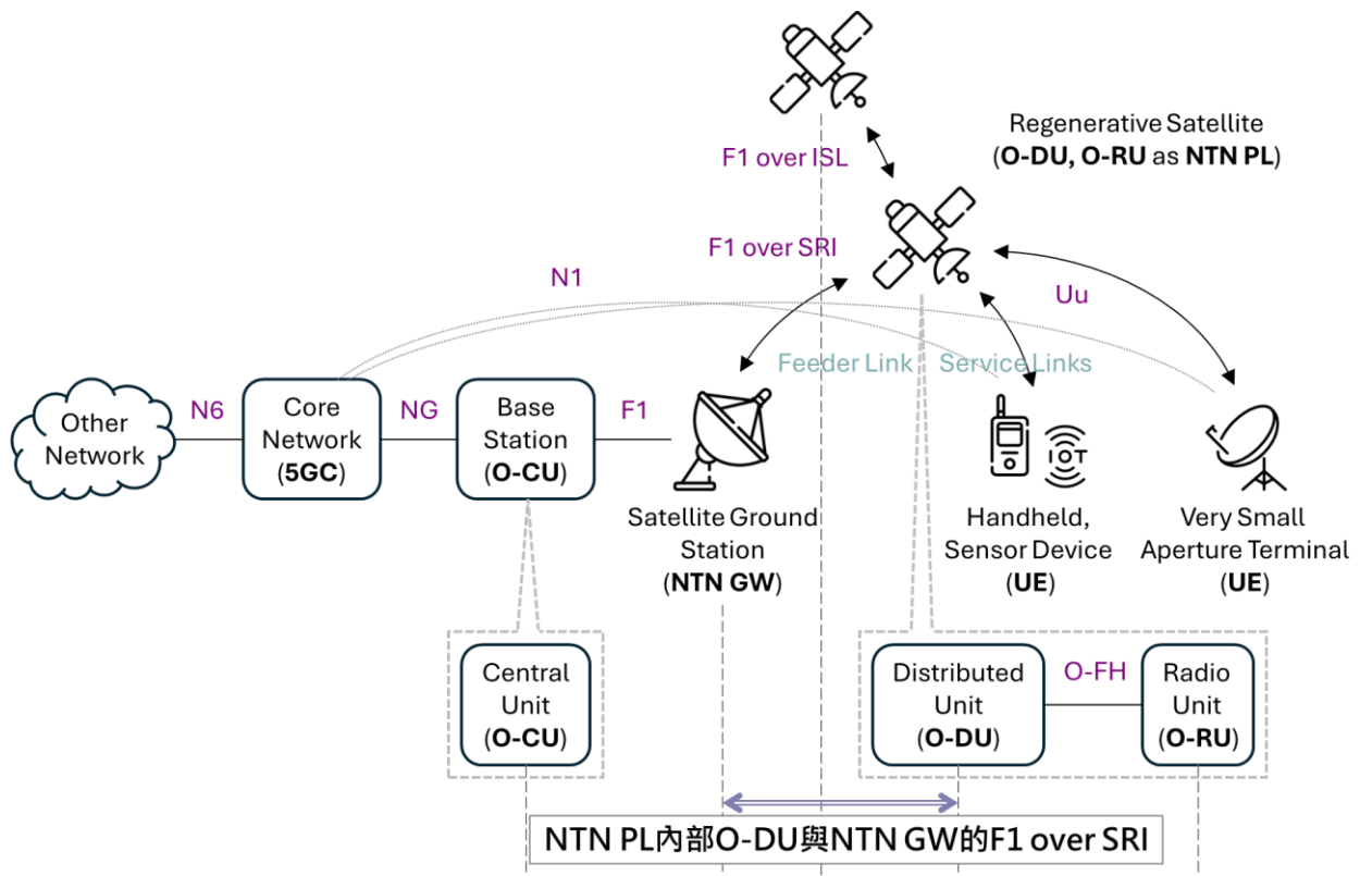
圖 61、3GPP NTN 再生型系統 O-RAN 的 NTN PL O-DU 與 NTN GW 的 F1 over SRI
