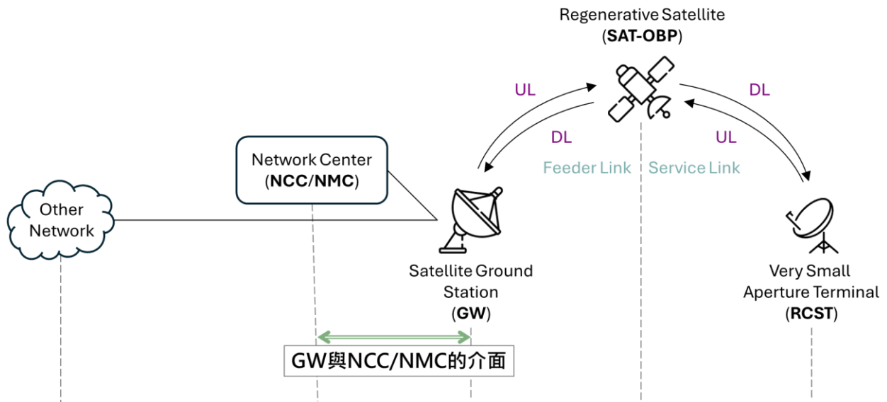
圖 39、DVB-S/RCS 再生型系統的 GW 與 NCC/NMC 的介面
