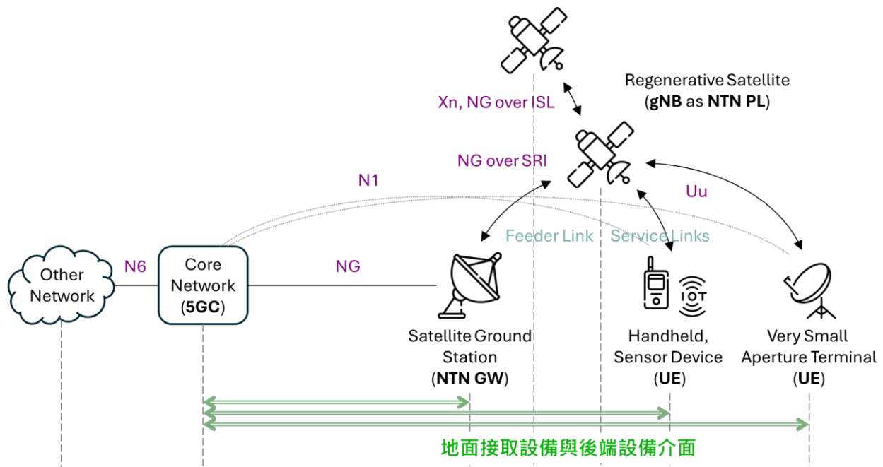
圖 20、3GPP NTN 再生型系統的地面接取設備與後端設備介面
