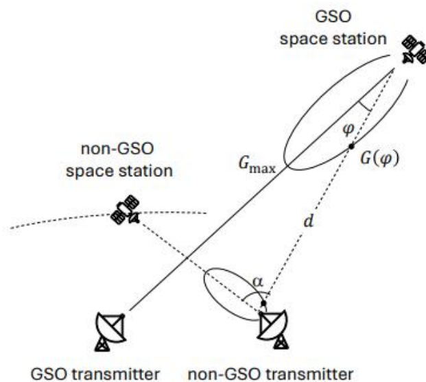
圖 32、規範上行方向干擾的 EPFD 示意
