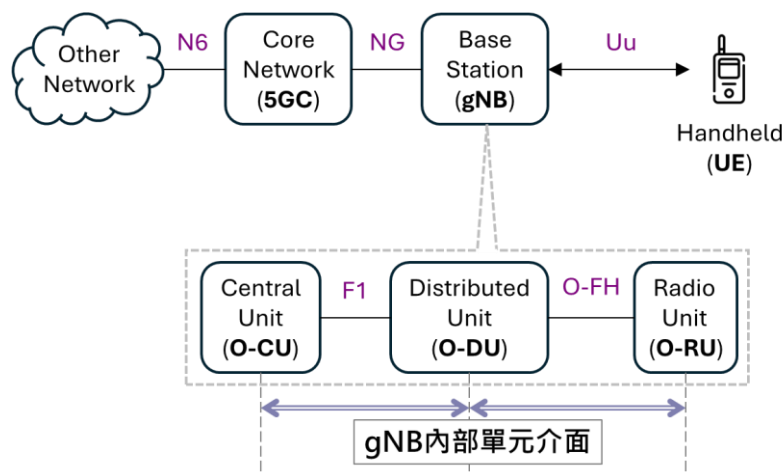
圖 57、3GPP 地面網路系統 O-RAN 單元介面
