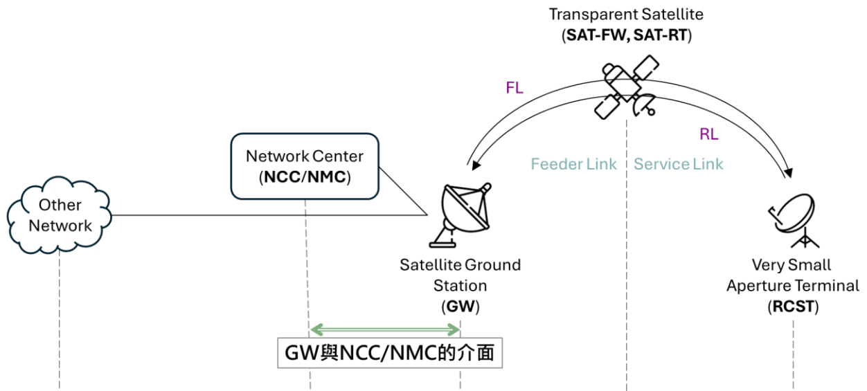
圖 38、DVB-S/RCS 通透型系統的 GW 與 NCC/NMC 的介面
