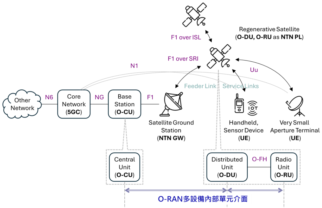
圖 30、3GPP NTN 再生型系統的 O-RAN 多設備內部單元介面
