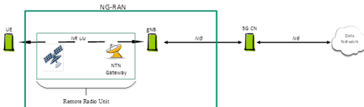
圖 7、3GPP NTN 通透型系統架構
