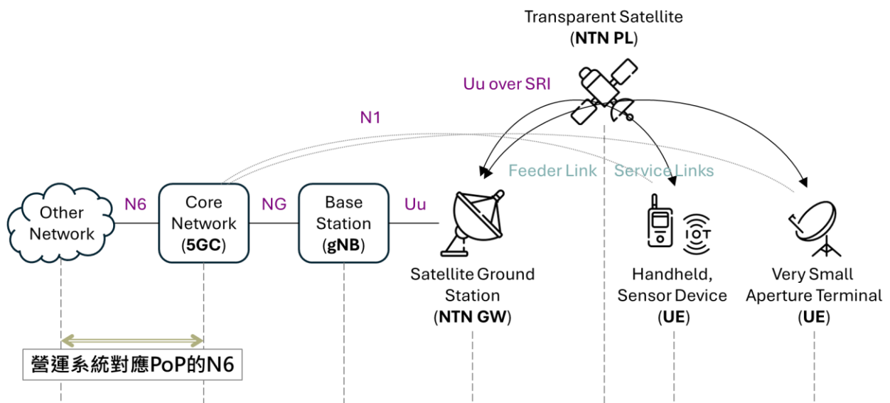
圖 36、3GPP NTN 通透型系統的營運系統對外介面
