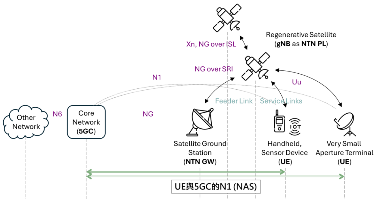
圖 44、3GPP NTN 再生型系統的 UE 與 5GC 的 N1 (NAS)
