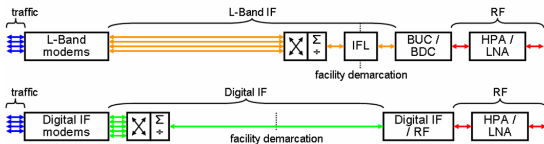
圖 51、傳統類比中頻 vs.數位中頻架構
