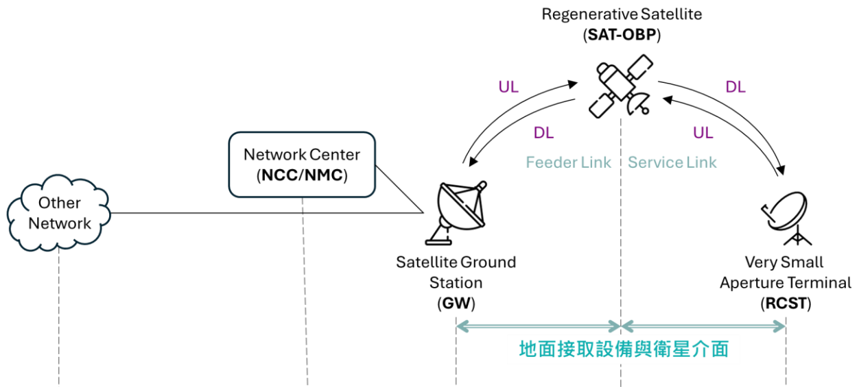
圖 22、DVB-S/RCS 再生型系統的地面接取設備與衛星介面
