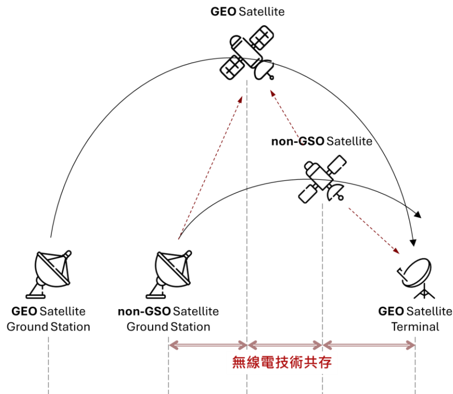
圖 12、GEO 與其他衛星系統的無線電技術共存
