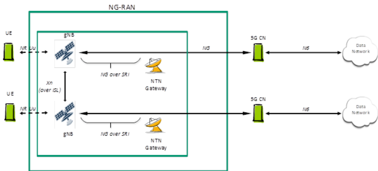
圖 9、3GPP NTN 再生型多衛星與多後端設備系統架構
