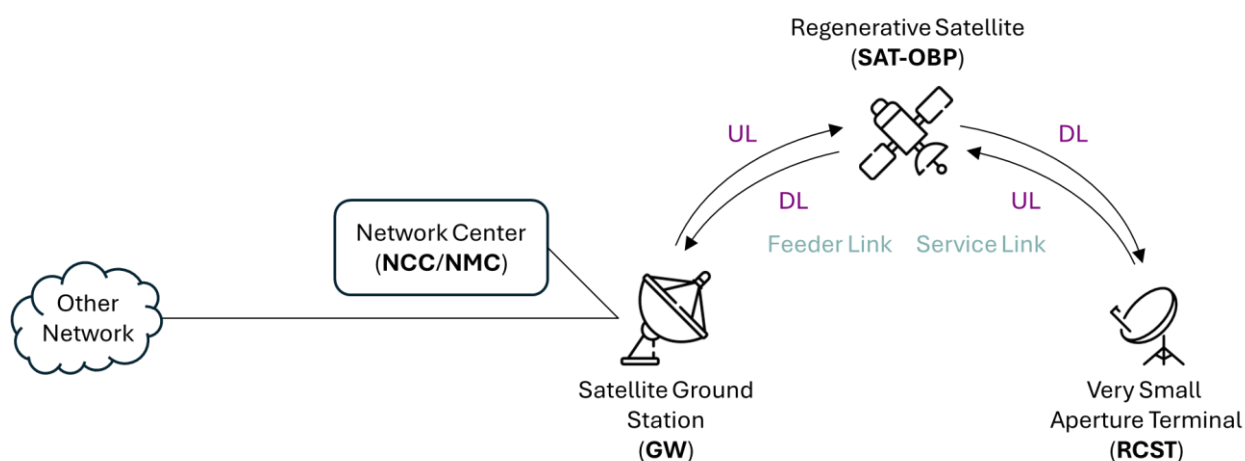
圖 6、DVB-S/RCS 再生型系統架構簡化示意
