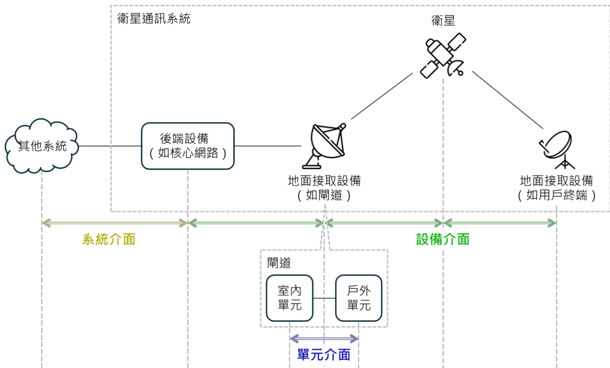
圖 2、衛星通訊系統中的介面類型範例
