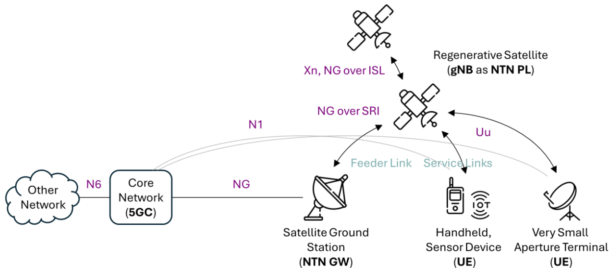
圖 11、3GPP NTN 再生型系統架構簡化示意
