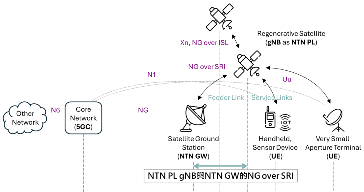
圖 49、3GPP NTN 再生型系統的 NTN PL gNB 與 NTN GW 的 NG over SRI
