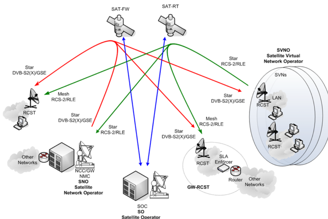
圖 3、DVB-S/RCS 通透型系統架構
