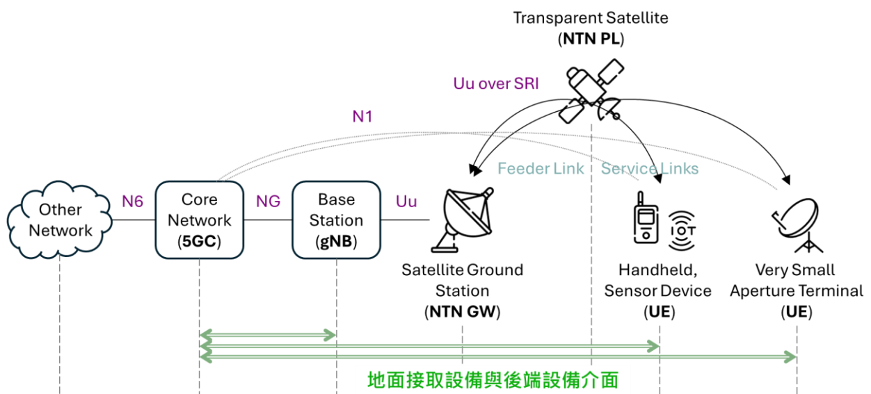
圖 19、3GPP NTN 通透型系統的地面接取設備與後端設備介面
