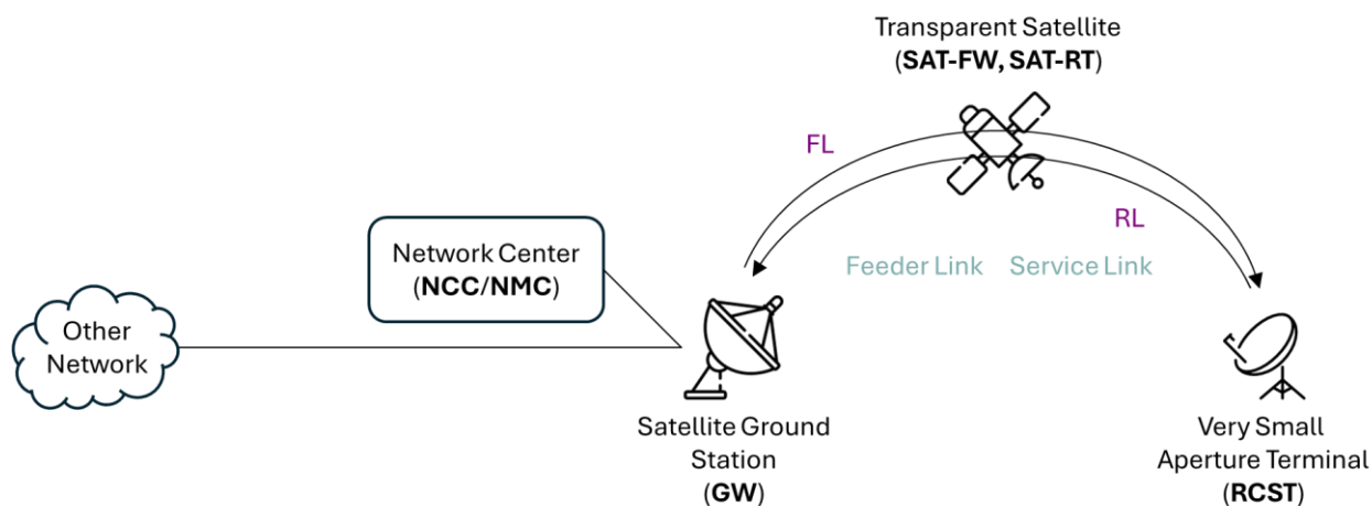
圖 5、DVB-S/RCS 通透型系統架構簡化示意
