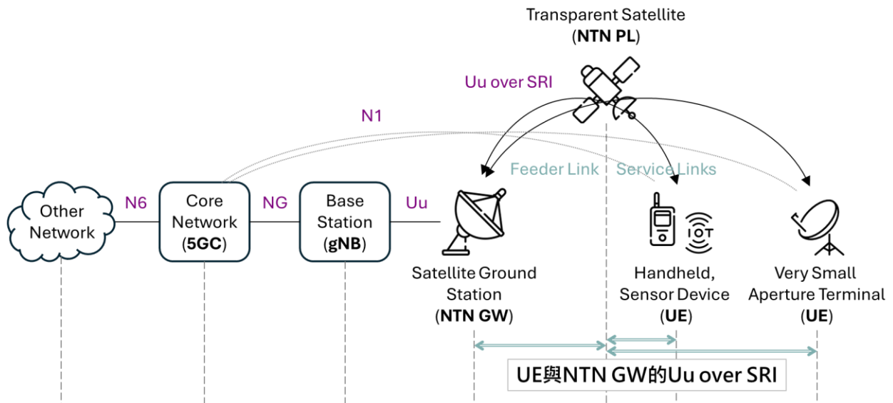
圖 47、3GPP NTN 通透型系統的 UE 與 NTN GW 的 Uu over SRI
