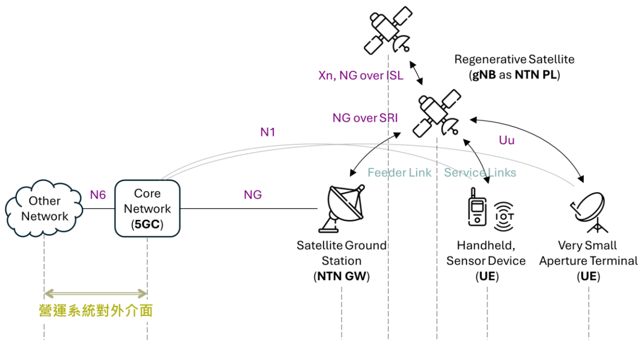
圖 16、3GPP NTN 再生型系統的營運系統對外介面
