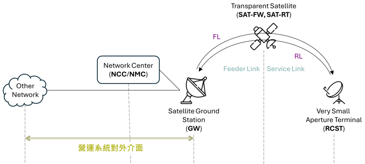
圖 13、DVB-S/RCS 通透型系統的營運系統對外介面
