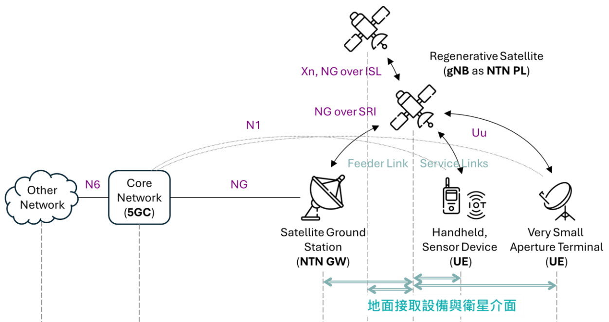
圖 24、3GPP NTN 再生型系統的地面接取設備與衛星介面
