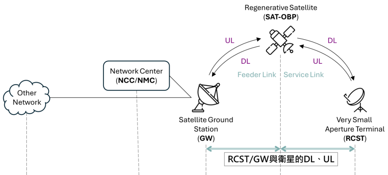
圖 46、DVB-S/RCS 再生型系統的 RCST/GW 與衛星的 DL、UL
