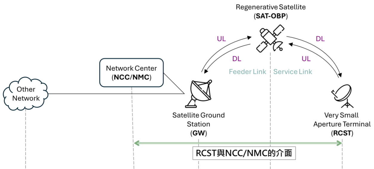
圖 41、DVB-S/RCS 再生型系統的 RCST 與 NCC/NMC 的介面
