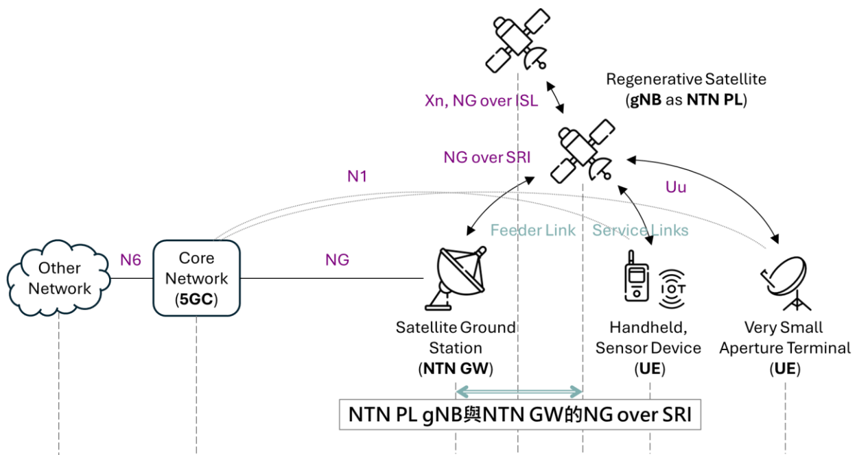
圖 58、3GPP NTN 通透型系統 O-RAN 的地面 gNB 內部單元的 O-FH 與 F1
