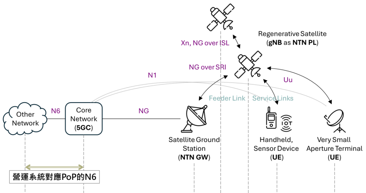
圖 37、3GPP NTN 再生型系統的營運系統對外介面
