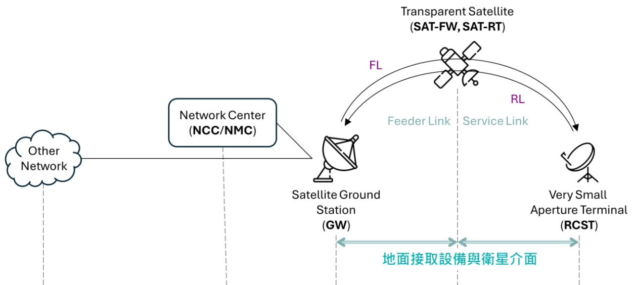
圖 21、DVB-S/RCS 通透型系統的地面接取設備與衛星介面
