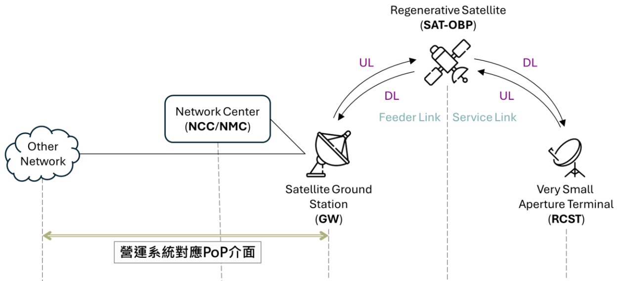
圖 35、DVB-S/RCS 再生型系統的營運系統對應 PoP 介面
