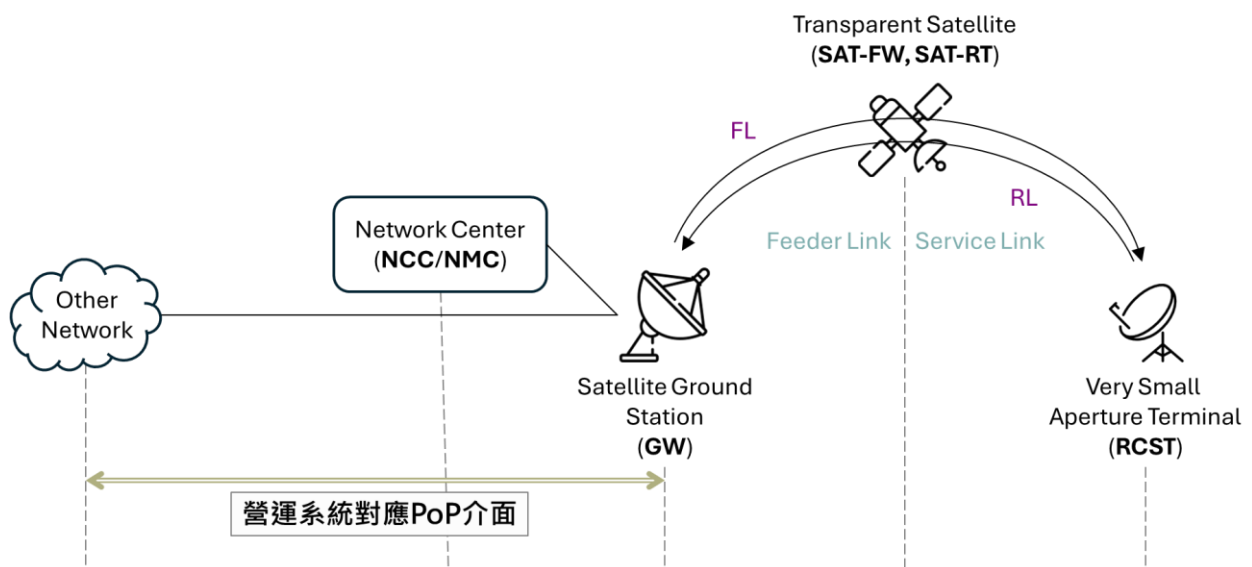
圖 34、DVB-S/RCS 通透型系統的營運系統對應 PoP 介面
