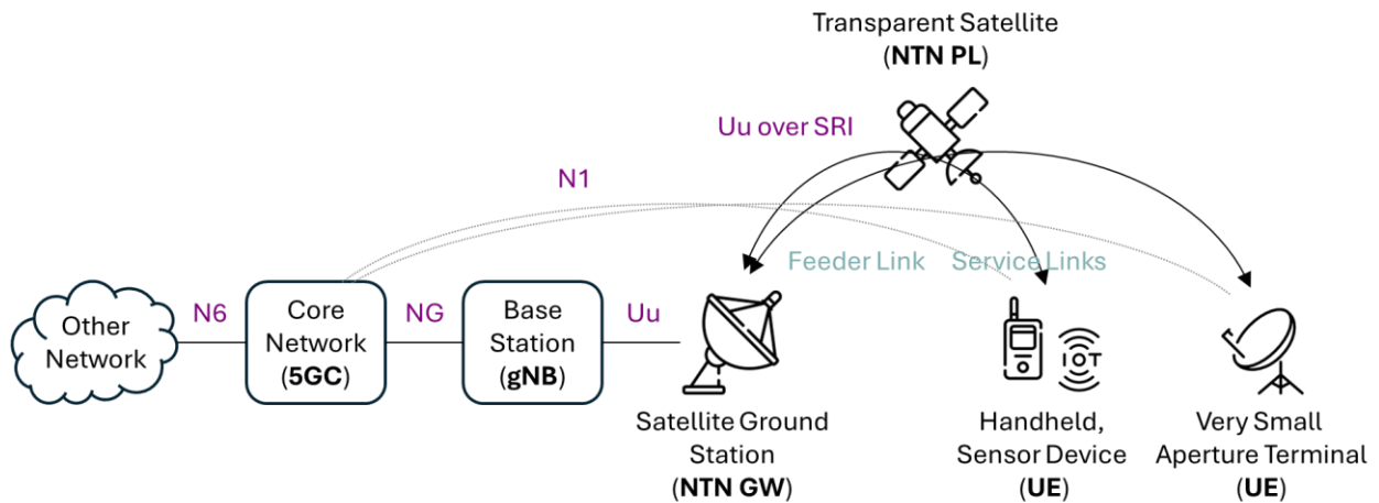
圖 10、3GPP NTN 通透型系統架構簡化示意
