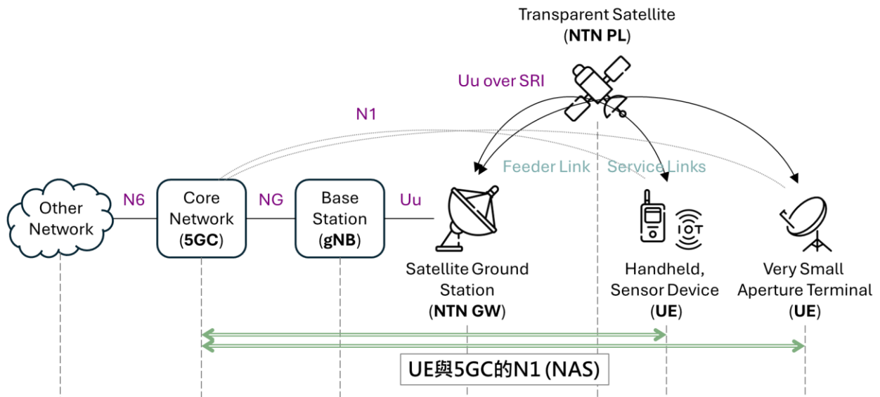
圖 43、3GPP NTN 通透型系統的 UE 與 5GC 的 N1 (NAS)
