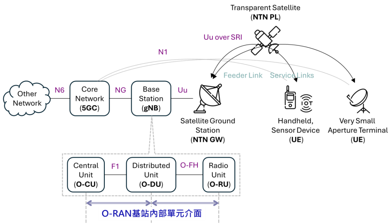
圖 29、3GPP NTN 通透型系統的 O-RAN 基站內部單元介面
