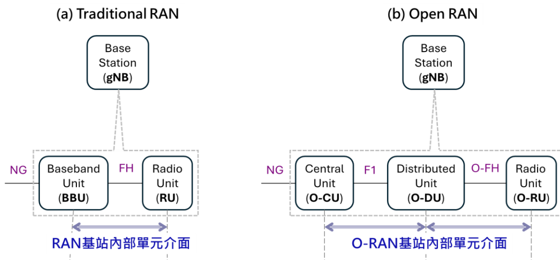
圖 28、3GPP RAN 基站內部單元介面 (a) 傳統 RAN 架構 (b) O-RAN 架構
